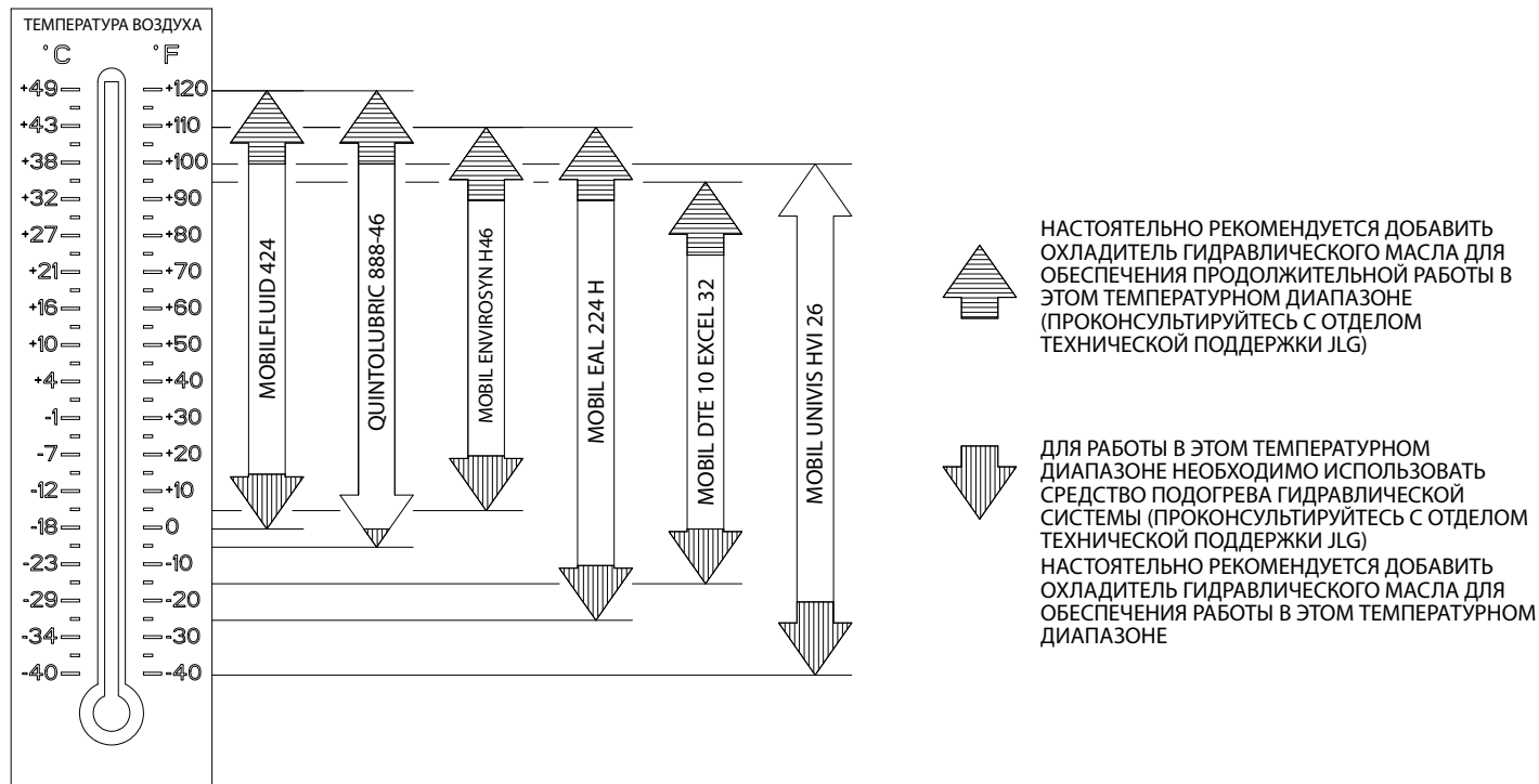
Рис. 7-1. Спецификации рабочей температуры гидравлической системы — лист 1 из 2
