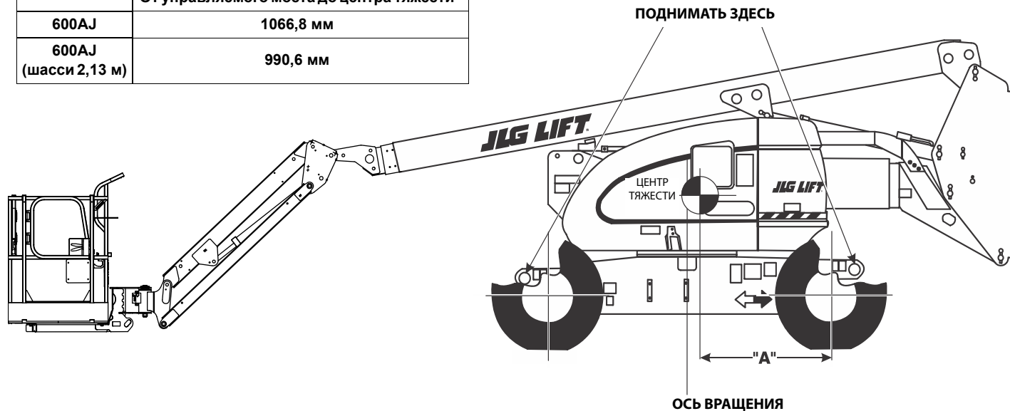
Рис. 4-7. Схема подъема
