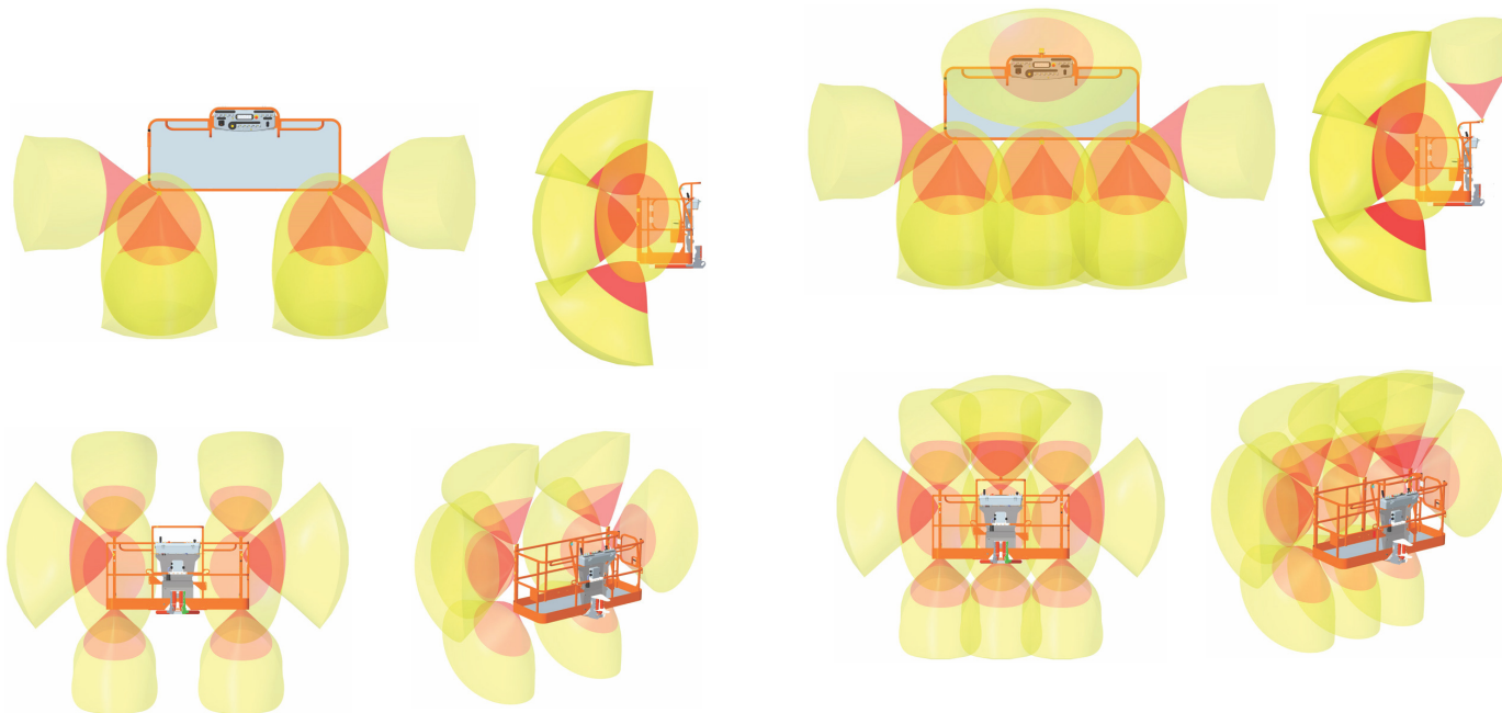
Уровень 2 (3 штанги)
