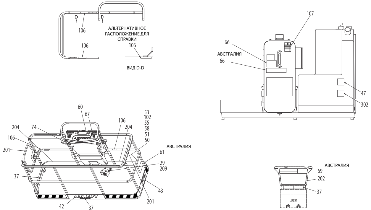
Рис. 4-10. Расположение наклеек модели 600AJ — лист 3 из 4
