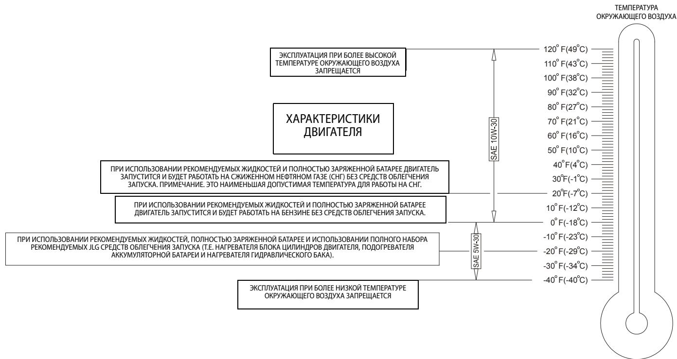
Рис. 7-5. Спецификации рабочей температуры гидравлической системы — лист 1 из 2
