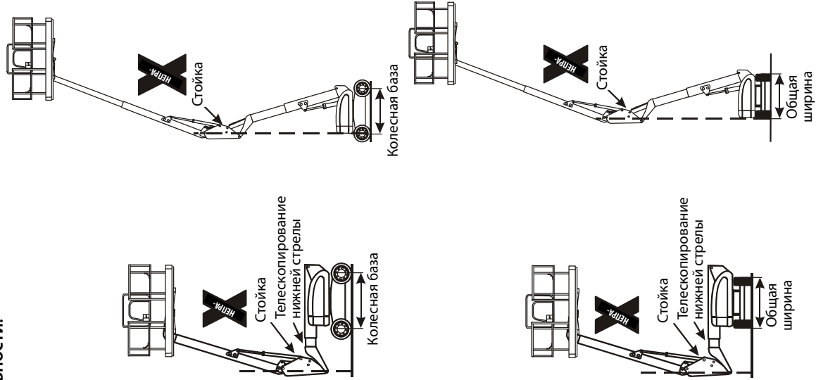
Рис. 4-5. Установка стоек стрелы — лист 2 из 2
