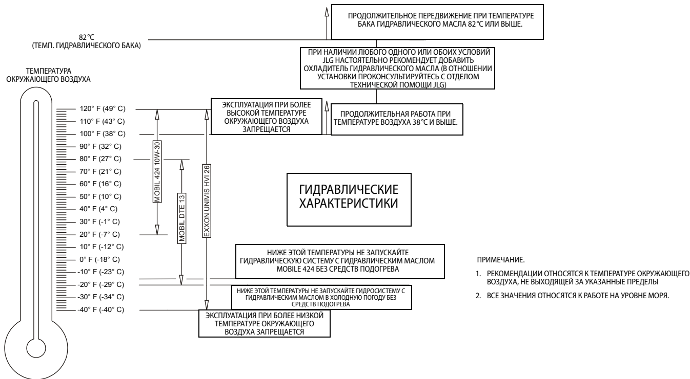
Рис. 7-6. Спецификации рабочей температуры гидравлической системы — лист 2 из 2
