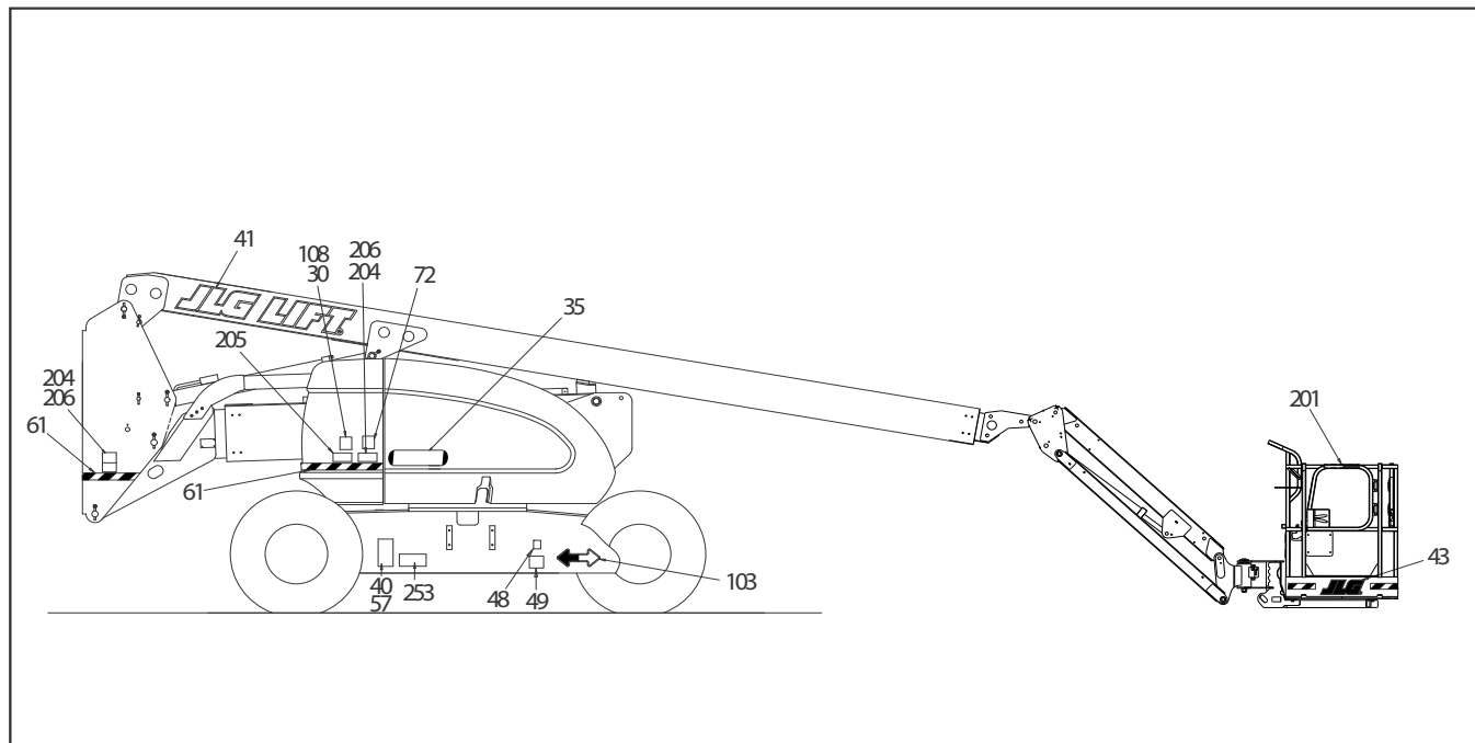
Рис. 4-9. Расположение наклеек модели 600AJ — лист 2 из 4
