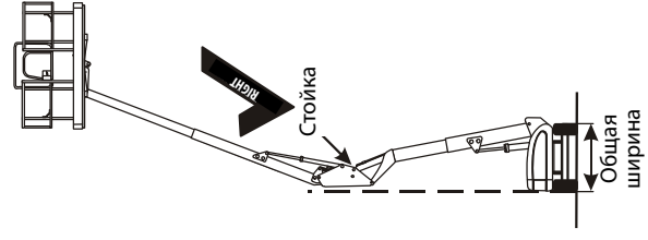
Рис. 4-4. Установка стоек стрелы — лист 1 из 2
