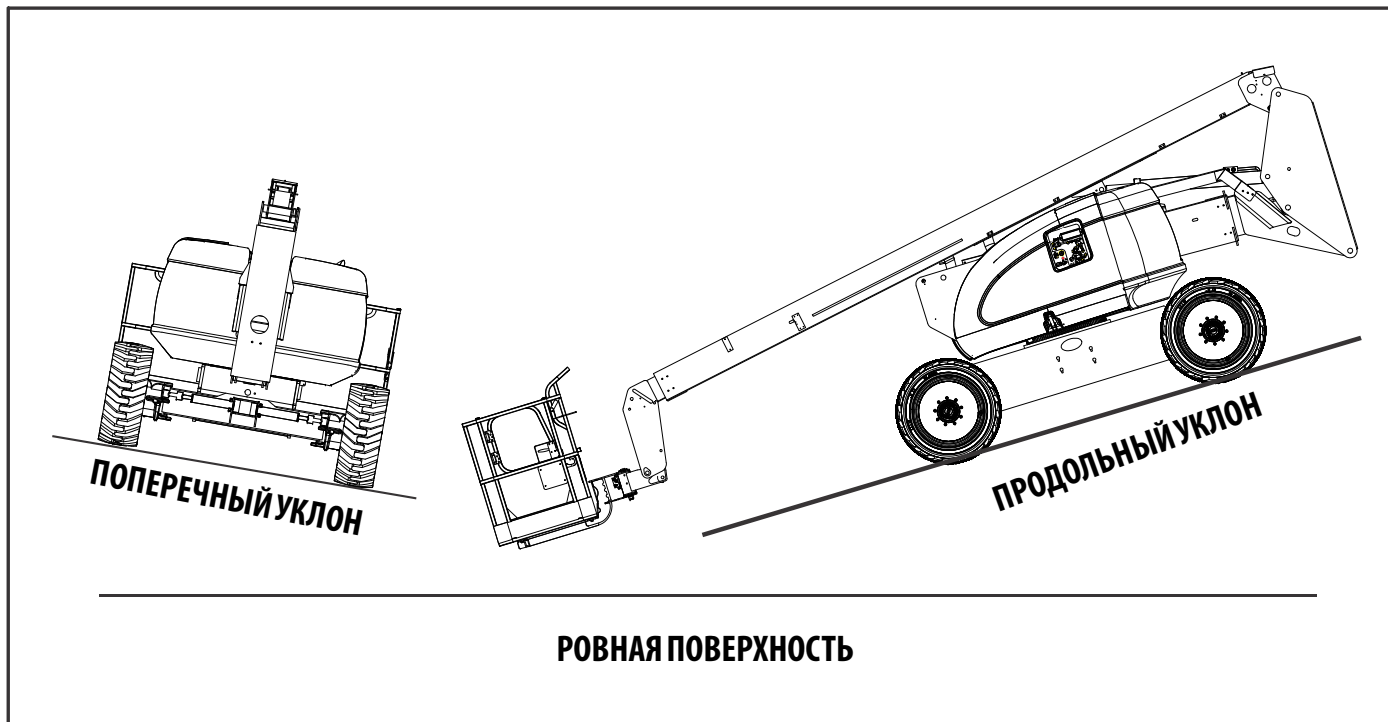
Рис. 4-2. Продольный и поперечный уклоны
