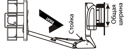
Рис. 4-4. Установка стоек стрелы — лист 1 из 2
