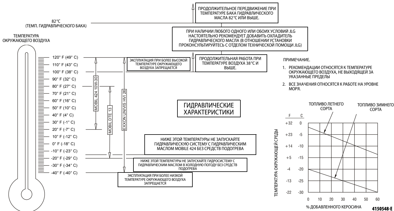
Рис. 7-4. Спецификации рабочей температуры гидравлических масел — Deutz — лист 2 из 2
